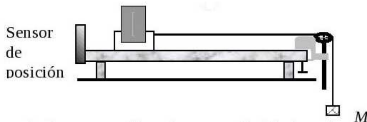
Figura 1: Dispositivo experimental para el estudio de la fuerza de rozamiento dinámica.
