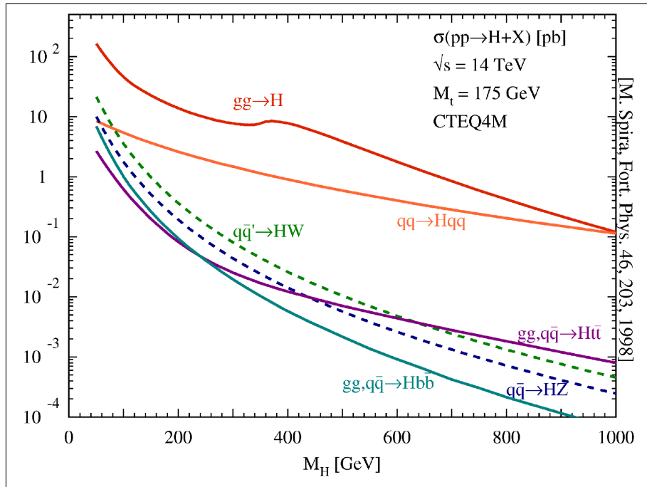
Figura 1: Canales de producción del Higgs en función de la masa del Higgs para el LHC.
