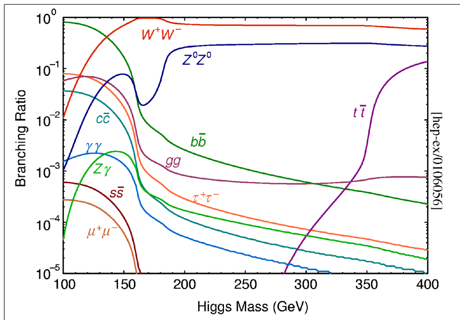
Figura 2: Ancho de los diferentes canales de decaimiento del Higgs en función de la masa del Higgs.
